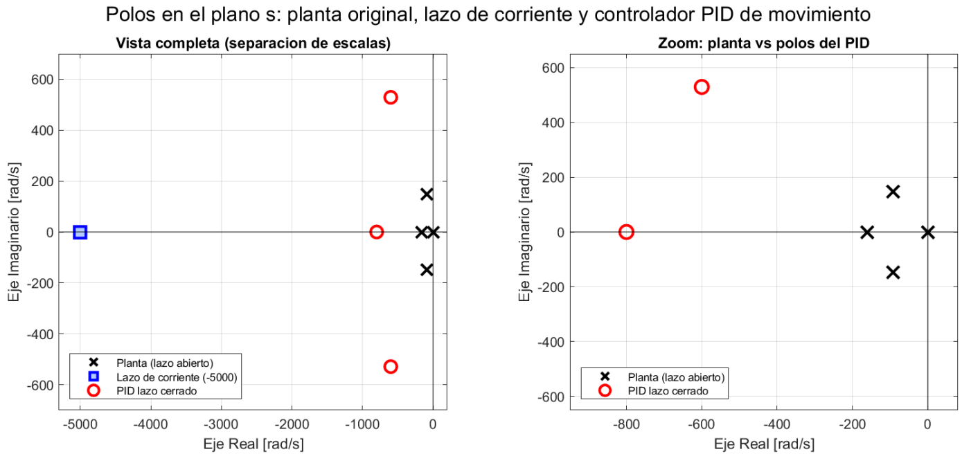
Fig. 38. Polos en el plano s : planta a lazo abierto (cruces), lazos de corriente (cuadrado, -5000 ) y polos de lazo cerrado del PID de movimiento (círculos, -800 y -600 \pm j529 ). Izquierda: vista completa (separación de escalas); derecha: zoom planta vs. PID.
