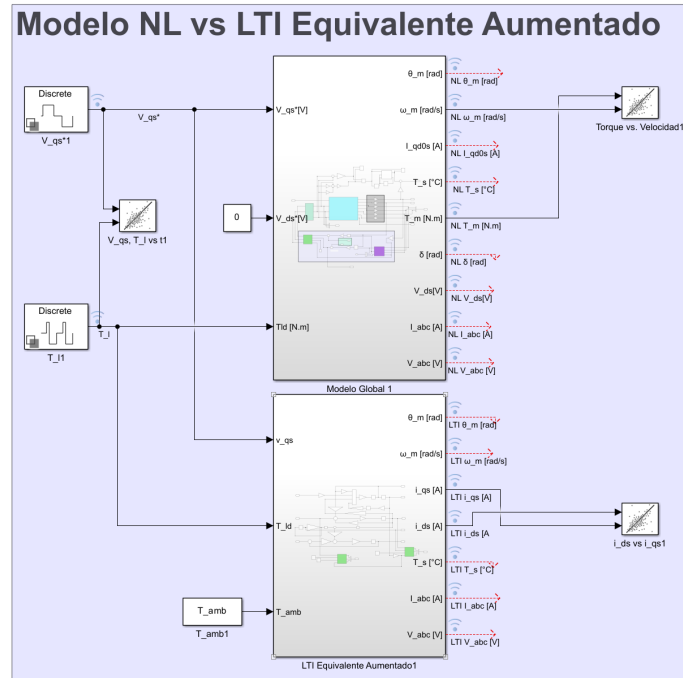
Fig. 15. Diagrama de bloques en Simulink: modelo NL desacoplado y LTI aumentado en paralelo frente al mismo V_{qs}^* consigna y Torque de Perturbacion.
