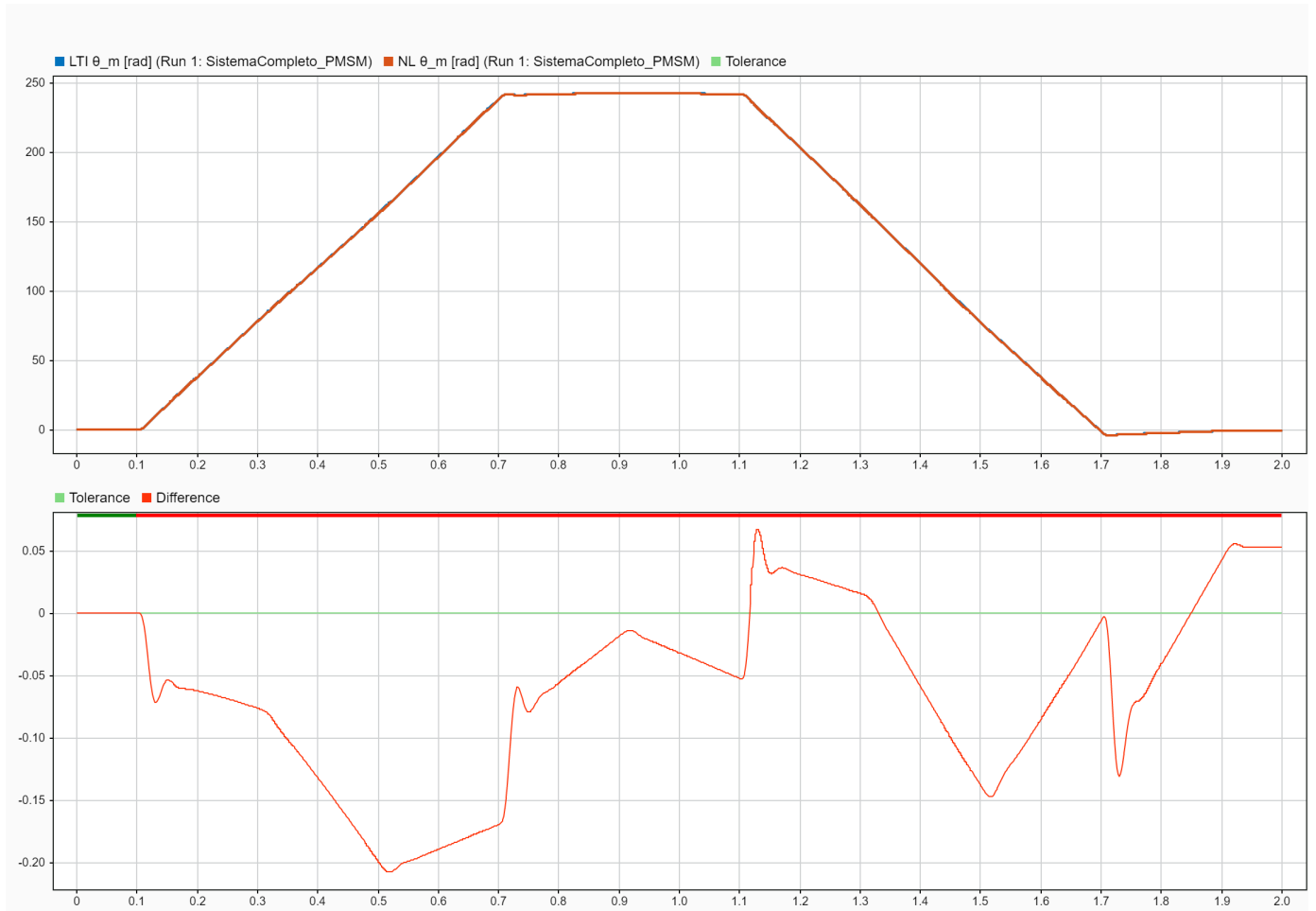
Fig. 17. Error de seguimiento en \theta_m(t) . Panel inferior: diferencia \theta_m^{NL} - \theta_m^{LTI} , acotada por debajo de 0,21 rad ( < 0,1\% de la excursión de 242 rad).
