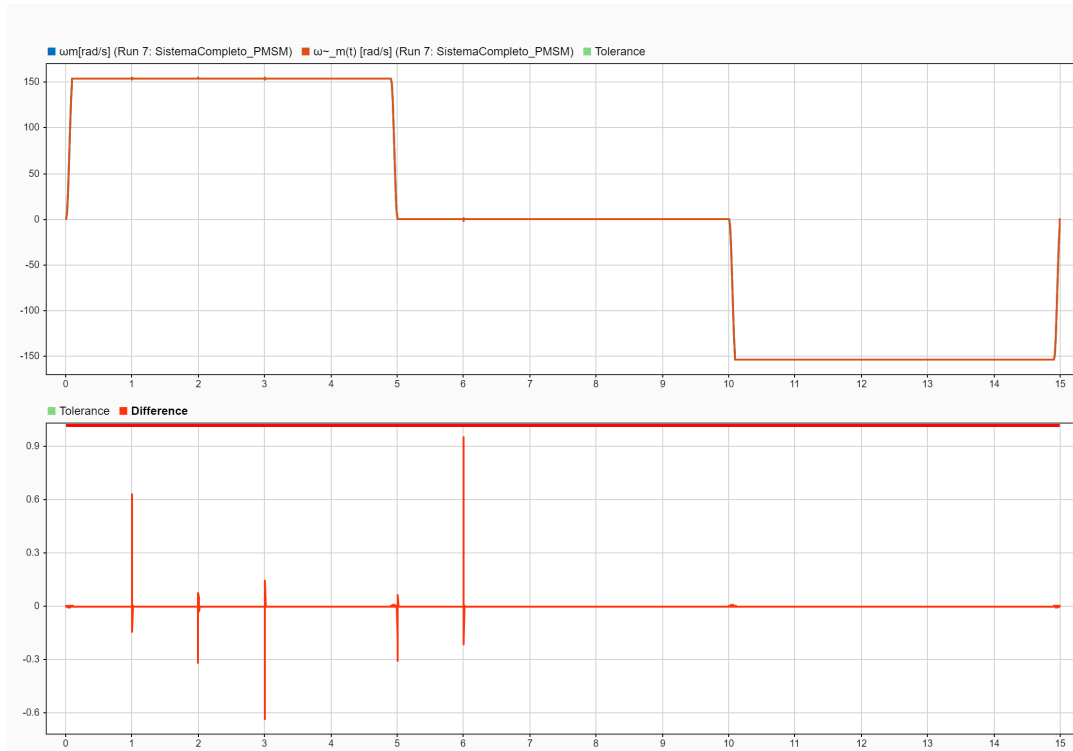
Fig. 55. Respuesta del observador aumentado con acción integral. Se observa la desaparición del error de offset en régimen permanente.
