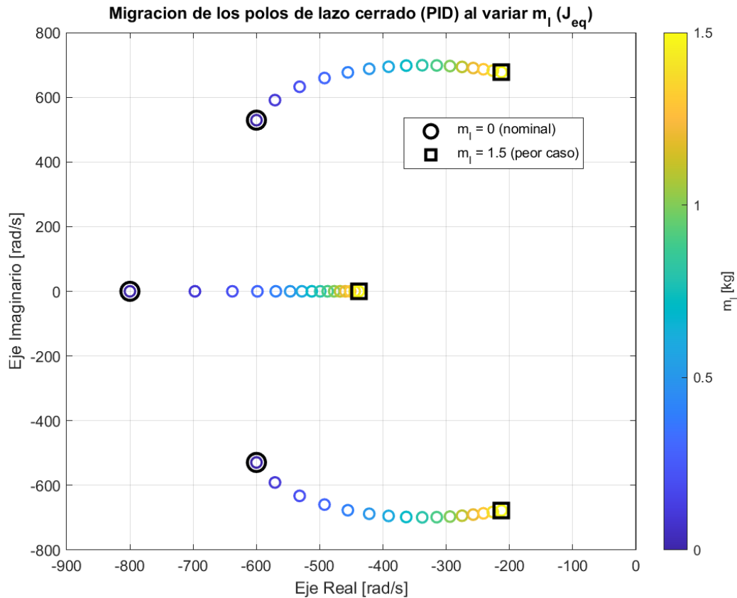
Fig. 39. Migración de los polos de lazo cerrado del PID al variar m_l de 0 a 1,5 kg con ganancias fijas (colorbar en m_l ). El nominal ( m_l = 0 ) se marca con círculo y el peor caso ( m_l = 1,5 ) con cuadrado.
