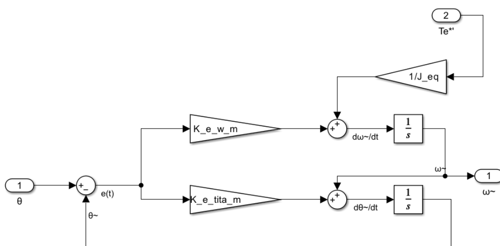
Fig. 40. Diagrama de bloques del observador de estados reducido
