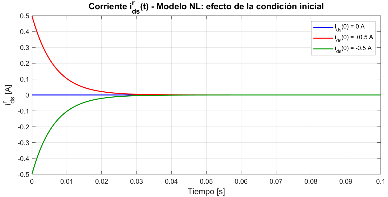
Fig. 27. Comparación de i_{ds}^r(t) para i_{ds}^r(0) \in \{0, +0,5, -0,5\} A: modelo NL.
