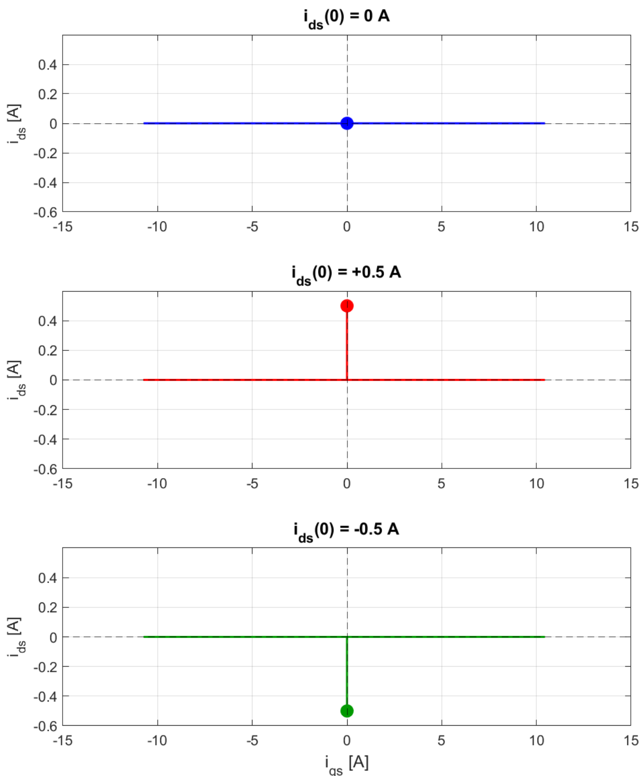
Fig. 29. Evolución de i_{ds}^r(t) frente a i_{qs}^r(t) para las tres condiciones iniciales i_{ds}^r(0) \in \{0, +0,5, -0,5\} A (modelo NL). Independientemente del valor inicial, la corriente de eje d converge al eje i_{ds}^r = 0 mientras i_{qs}^r desarrolla el torque, evidenciando el desacople efectivo entre ambos ejes.
