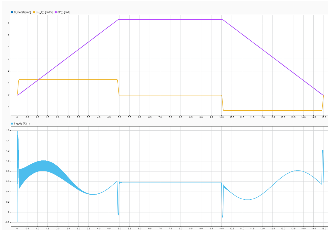
Fig. 60. Arriba Posición y Velocidad, debajo corriente en eje en cuadratura. Finalmente se consigue un rendimiento satisfactorio y cumplimiento con las demás condiciones de operación al mismo tiempo. ( T_{ld} = 5 [Nm], \omega_n = 12000 [rad/s])
