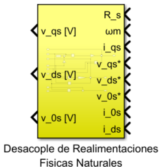
Fig. 32. Bloque (subsistema) equivalente del desacoplamiento de retroalimentaciones físicas naturales.
