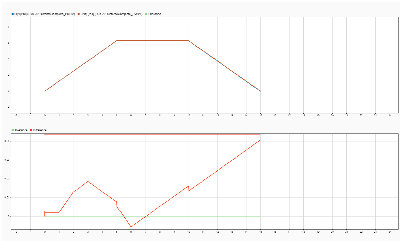
Fig. 48. Seguimiento de posición con saturación de tensión del inversor en 39,19 V.
