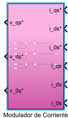
Fig. 36. Subsistema del modulador (lazo proporcional) de corrientes.
