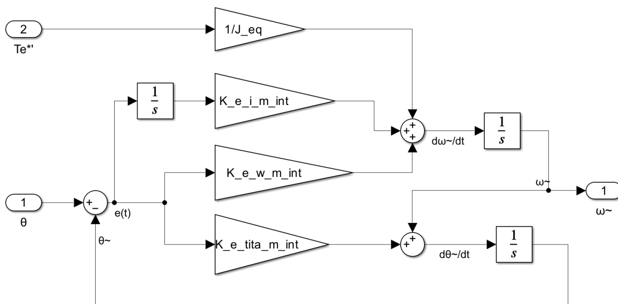
Fig. 54. Diagrama de bloques del observador mecánico aumentado con acción integral implementado en Simulink. El error de posición e_{\theta}(t) = \theta_m(t) - \hat{\theta}_m(t) alimenta tanto las ramas proporcionales como la rama integral, cuya salida corrige la dinámica de \hat{\omega}_m(t) para eliminar el error estacionario de estimación.
