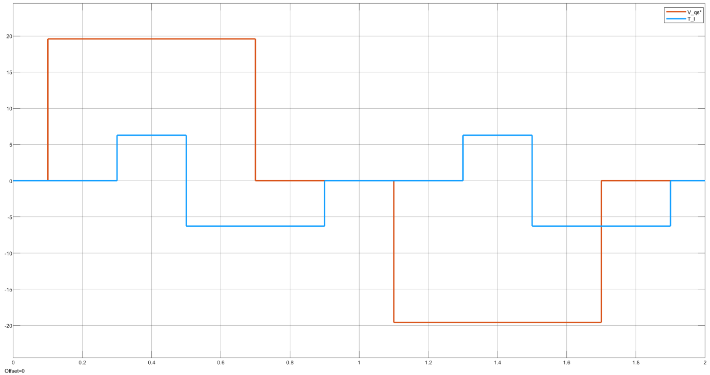
Fig. 14. Señales de excitación: consigna de tensión v_{qs}^*(t) y torque de carga T_{ld}(t) .
