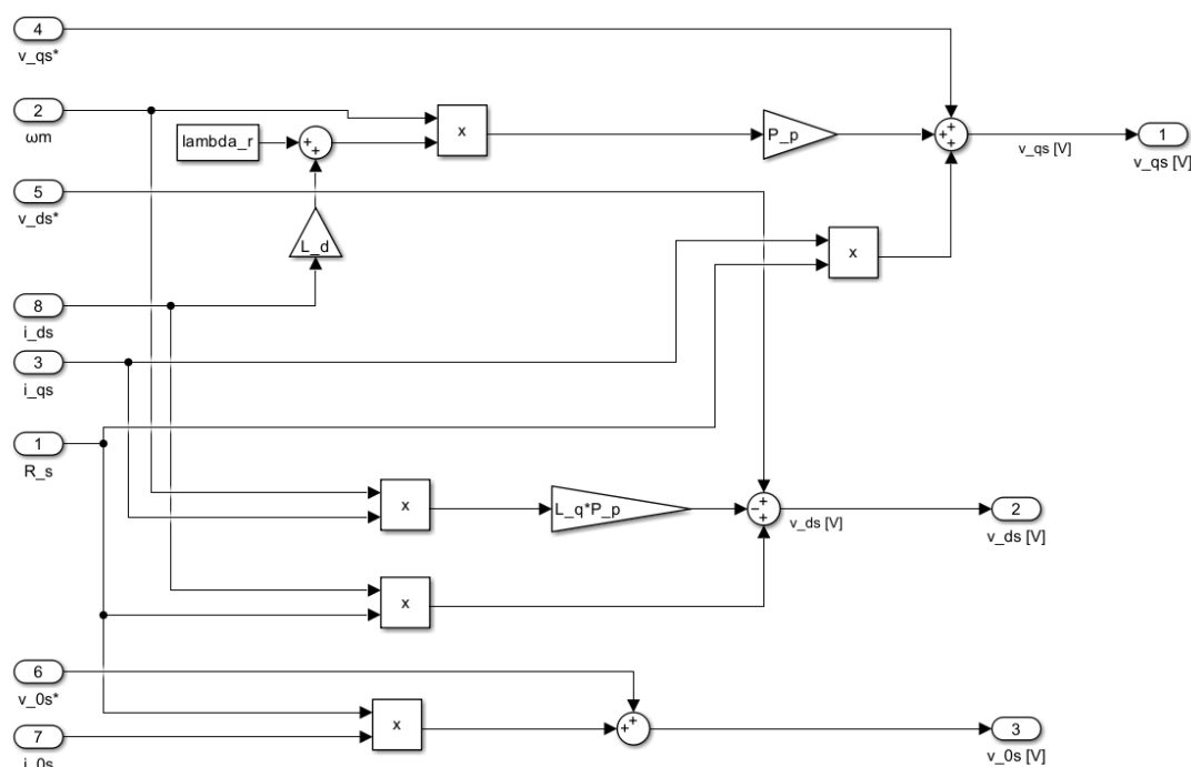
Fig. 31. Implementación en Simulink del desacoplamiento de las retroalimentaciones físicas naturales: las tensiones de referencia v_{qd0s}^{r*} cancelan las caídas resistivas R_s(T_s^\circ) i , la fuerza contraelectromotriz y los acoplamientos cruzados entre los ejes q y d .
