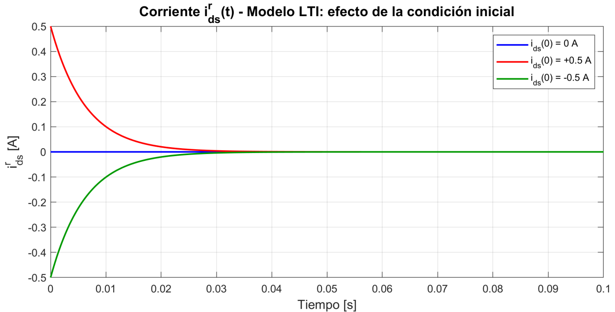
Fig. 28. Comparación de i_{ds}^r(t) para i_{ds}^r(0) \in \{0, +0,5, -0,5\} A: modelo LTI.
