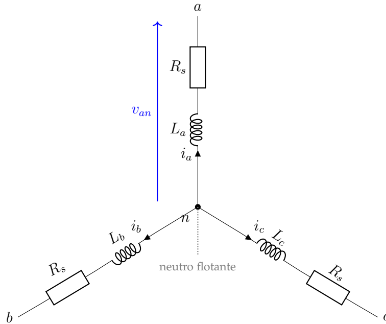
Fig. 2. Estator trifásico conectado en estrella con neutro flotante. Al no existir conductor de retorno externo, la Ley de Corrientes de Kirchhoff aplicada en el nodo neutro impone i_a + i_b + i_c = 0 , por lo que la componente homopolar de corriente resulta nula: i_{0s}(t) \equiv 0 .
