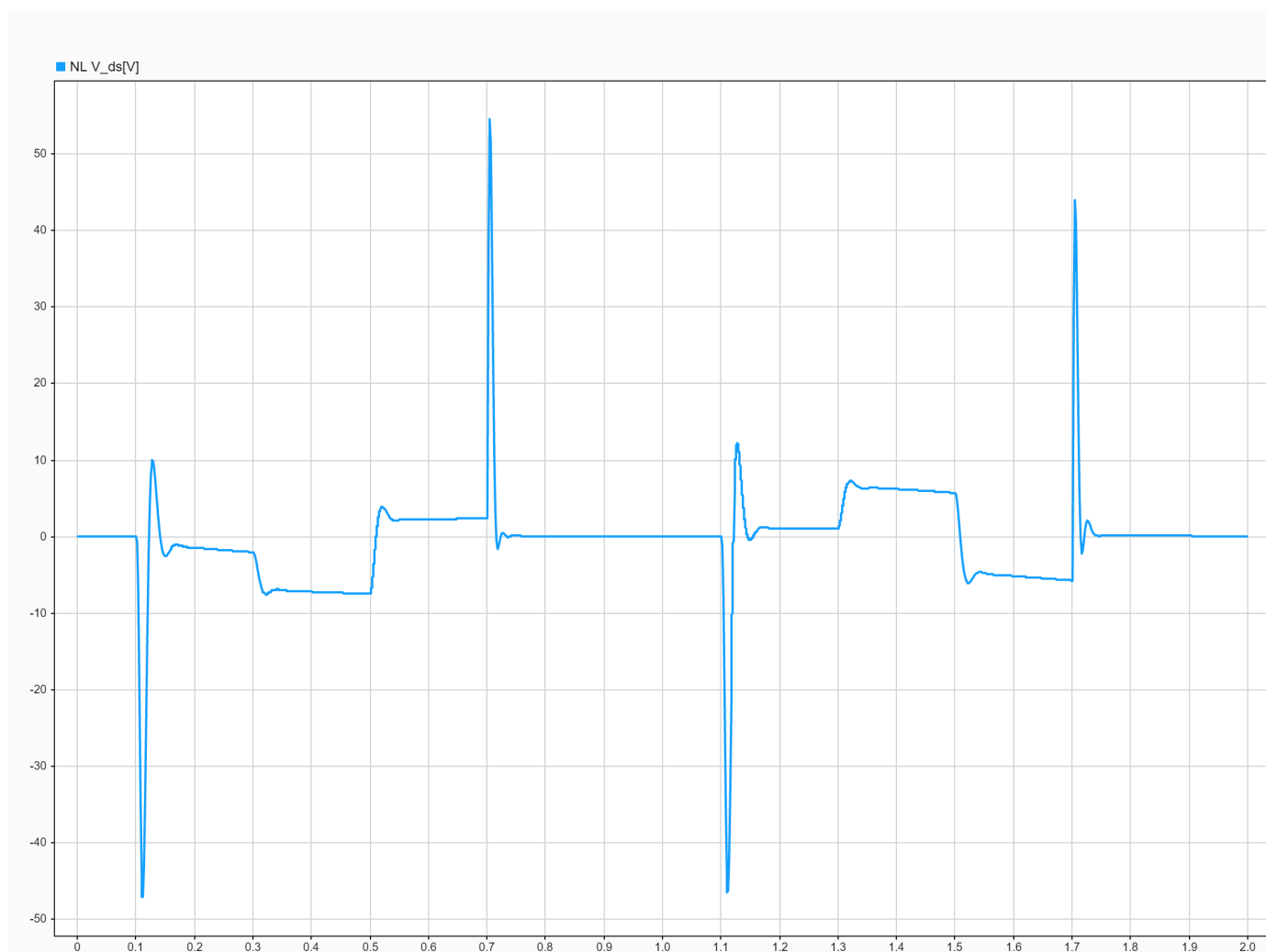
Fig. 23. Tensión v_{ds} vs t : modelo NL ( i_{ds}^r(0) = 0 A).
