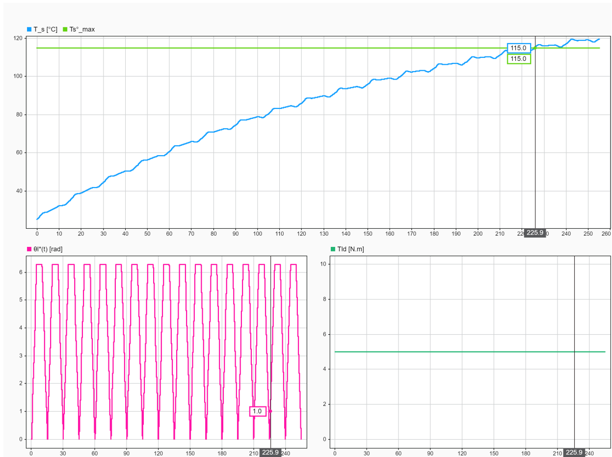
Fig. 56. Evolución de la temperatura del bobinado T_s^{\circ}(t) bajo operación repetitiva, considerando T_{amb} = 25^{\circ}\text{C} , T_{Ld} = 5 \text{ Nm} y la consigna trapezoidal de posición utilizada en el trabajo. Se observa que la temperatura supera el límite admisible T_{s,\max} = 115^{\circ}\text{C} a los 225.9 s.
