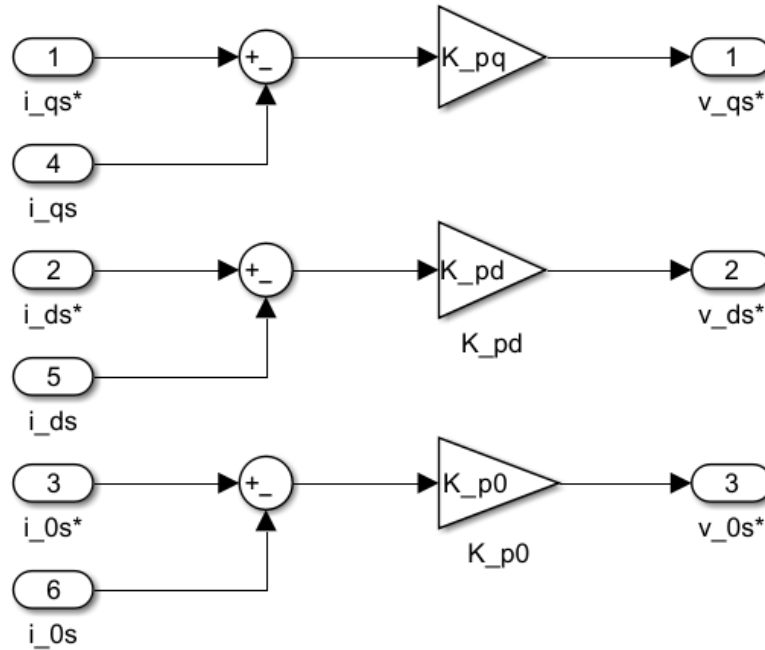
Fig. 35. Lazos de control de corriente i_{qd0s}^T con acción proporcional, ubicando los polos del lazo interno en p_i = -5000 rad/s.
