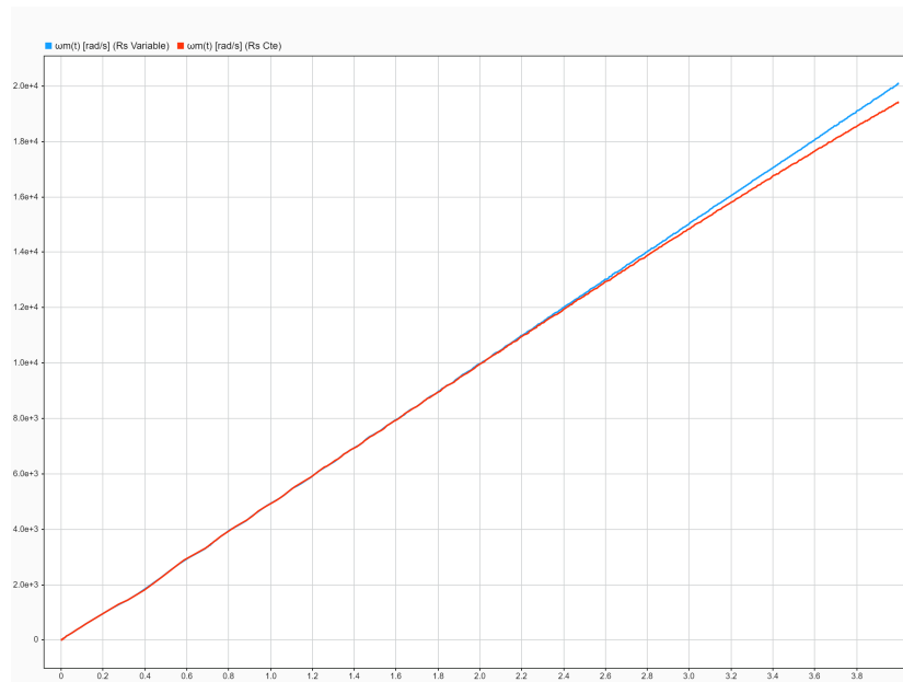
Fig. 34. Comportamiento de la velocidad angular mecánica ( \omega_m(t) ) en [rad/s] en función del tiempo. Se comparan las respuestas con resistencia estática constante (RS Cte., línea roja) y con resistencia estática variable (RS Variable, línea azul).
