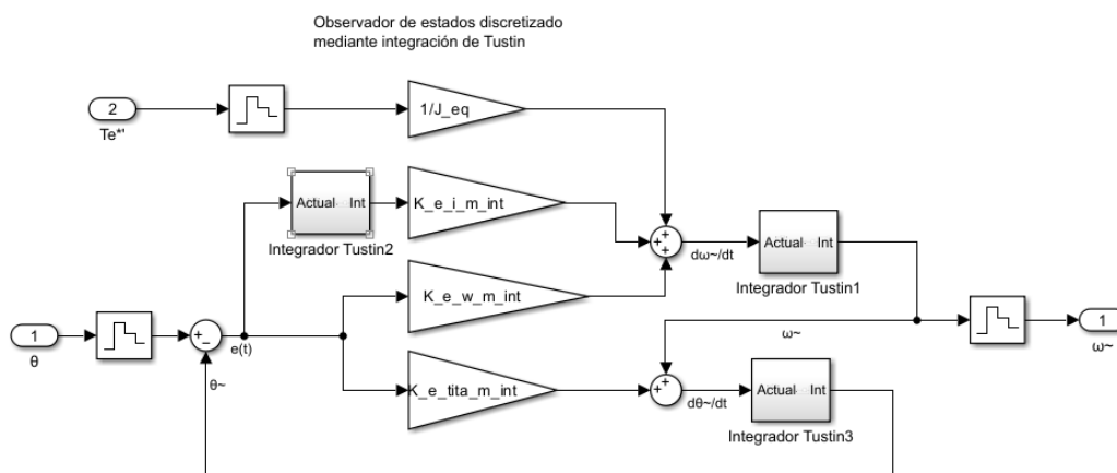
Fig. 61. Diagrama de bloques del observador discretizado. (Incorporación de ZOH, y reemplazo de integradores continuos por Integradores de Tustin)
