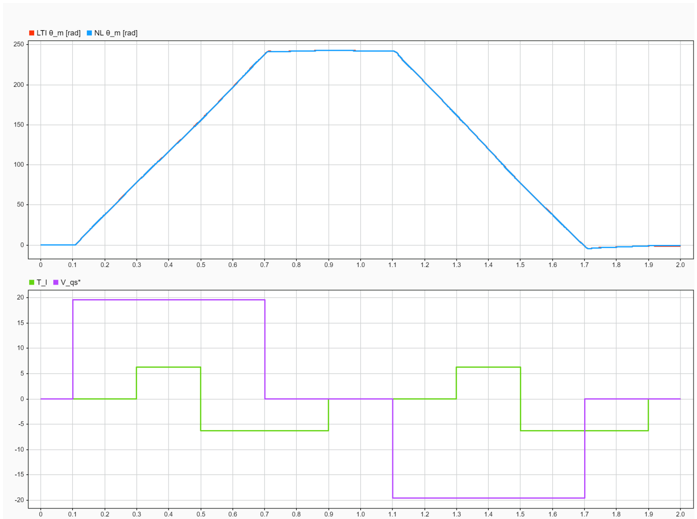
Fig. 16. Posición angular \theta_m(t) : comparación NL (azul) vs LTI aumentado (rojo). Panel inferior: señales de excitación (torque de carga T_l y consigna v_{qs}^* ).
