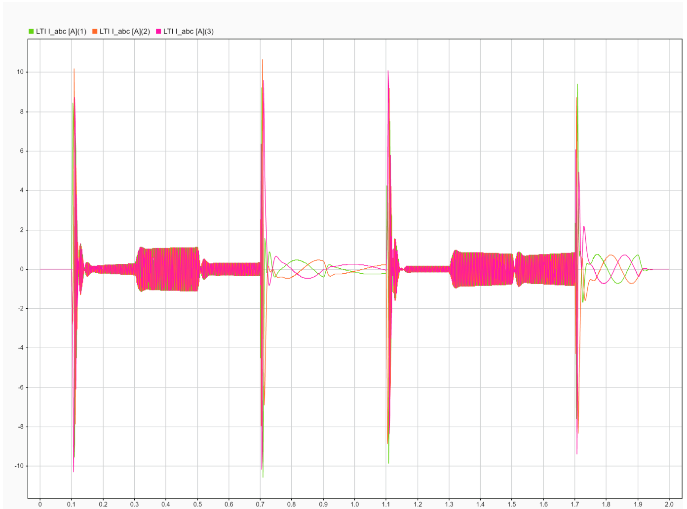
Fig. 24. Corrientes de fase i_a , i_b , i_c obtenidas por Transformación Inversa de Park (modelo NL, i_{ds}^r(0) = 0 A).
