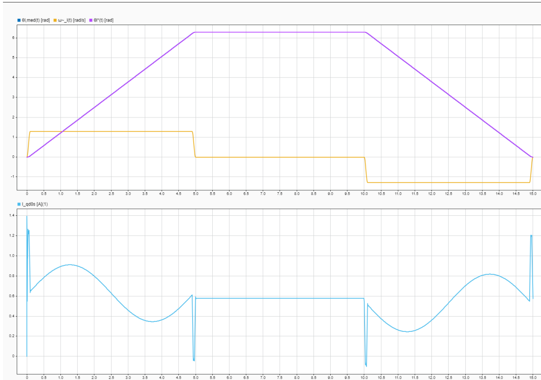
Fig. 58. Arriba Posición y Velocidad, debajo corriente en eje en cuadratura. Puede verse como ya el accionamiento sigue con éxito la consigna de solicitada sin oscilaciones producidas por los retardos de los sensores. ( T_{ld} = 5 [Nm])
