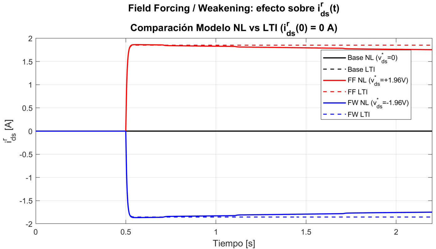
Fig. 30. Efecto del field forcing ( v_{ds}^* = +1,96 V) y field weakening ( v_{ds}^* = -1,96 V) sobre i_{ds}^r(t) , comparado con el caso base ( v_{ds}^* = 0 ).
